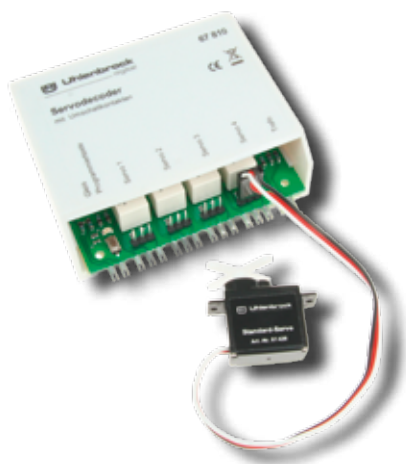
An einen Servodecoder 67810 können bis zu vier Servos angeschlossen werden.
