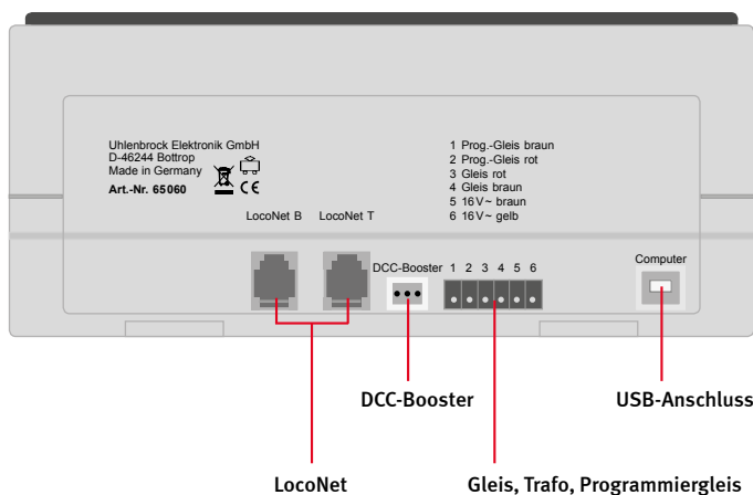
Die Anschlüsse der Intellibox Basic
