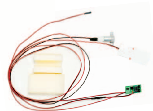
159012 Antriebsset für Windenergieanlage für Art.-Nr. 159005, bestehend aus Motor, Elektronik, Verkabelung und Dämmschaumstoff Set of electronic gearing for the wind energy plant for Art.-Nr. 159005, composed of motor, electronic gearing, cabling and foam
