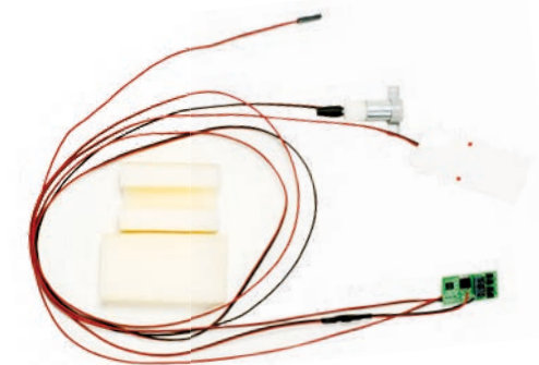
159012 Antriebsset für Windenergieanlage für Art.-Nr. 159005, bestehend aus Motor, Elektronik, Verkabelung und Dämmschaumstoff Set of electronic gearing for the wind energy plant for Art.-Nr. 159005, composed of motor, electronic gearing, cabling and foam
