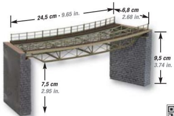
Brückenfahrbahn, gebogen, mit Brückenköpfen Bridge Deck, curved, incl. bridge heads
