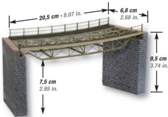
Brückenfahrbahn, gebogen, mit Brückenköpfen Bridge Deck, curved, incl. bridge heads
